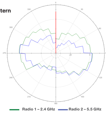
H-Plane Pattern
